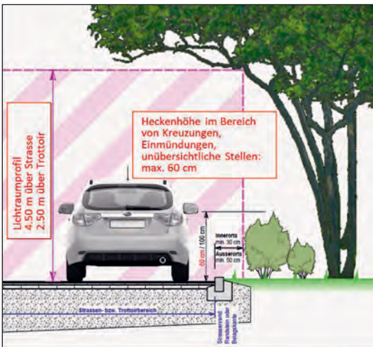
Lichtraumprofil
